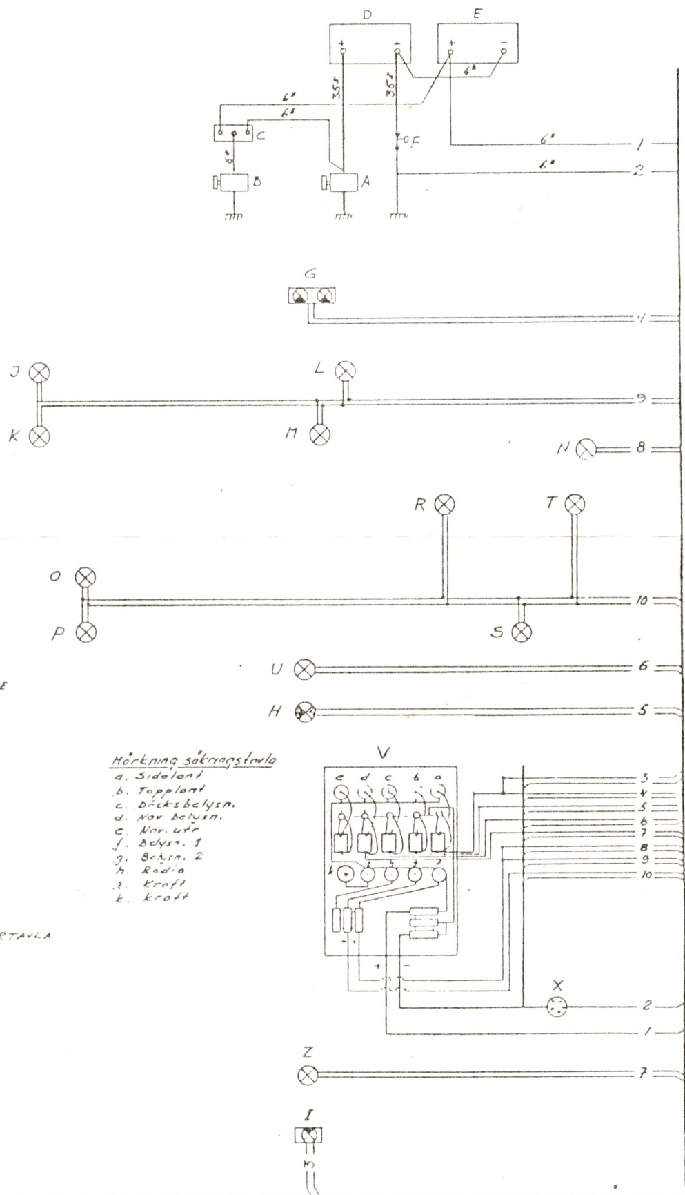
ELSCHEMA SCANMAR 33
